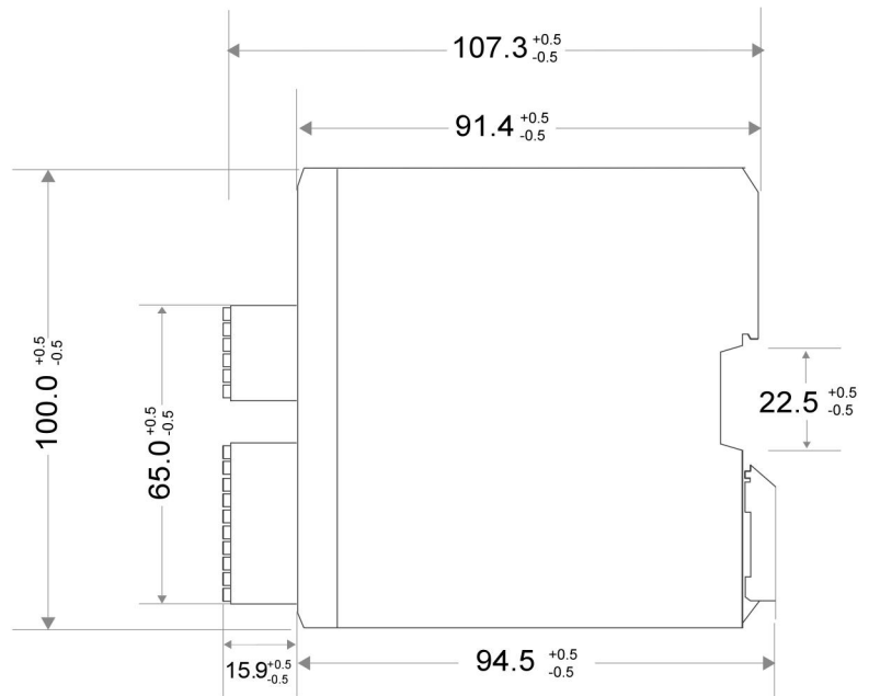
侧视图
